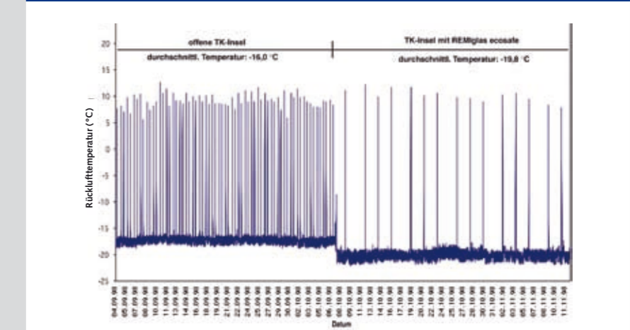
Energieverbrauch TK-Insel
