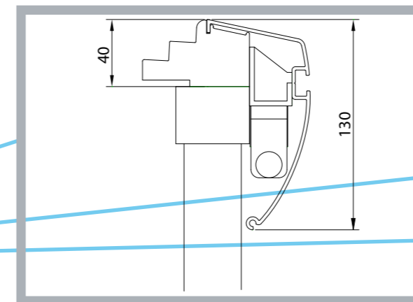
Handlauf mit Beleuchtung (130 mm)
