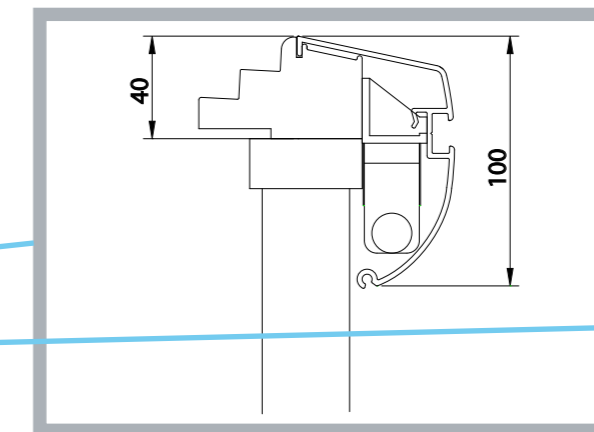
Handlauf mit Beleuchtung (100 mm)
